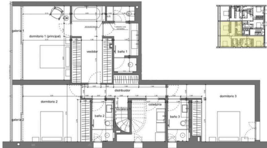
Planta 2
